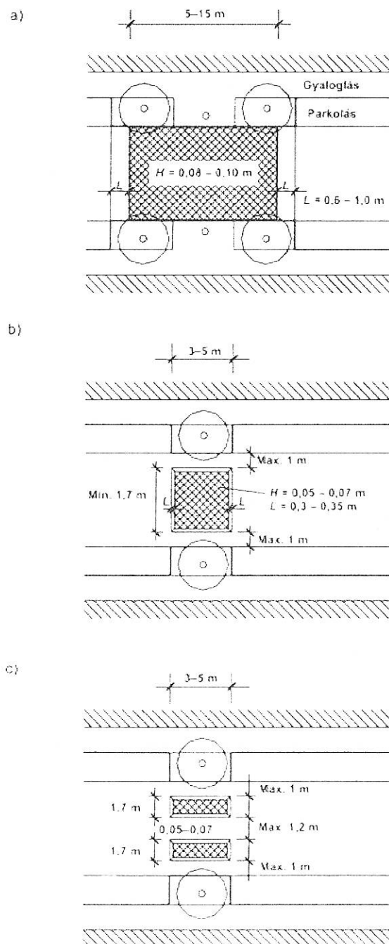
16. ábra - Szintemelések főbb méretei a) Részbeni szintemelés b) Egyes lemezszintemelés c) Osztott lemezszintemelés
